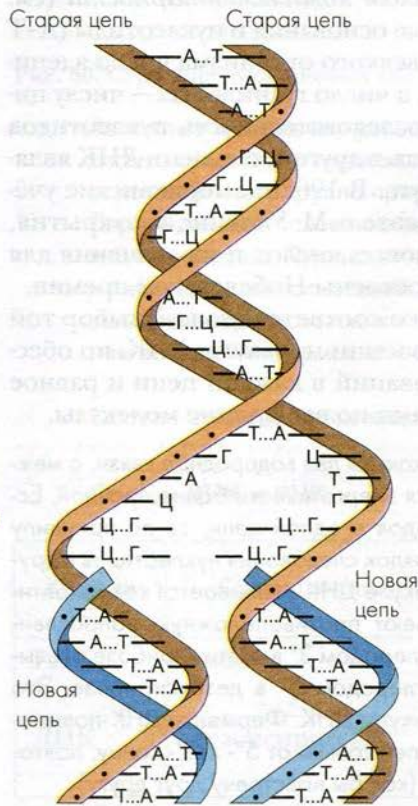
Рис. 61. Репликация ДНК
