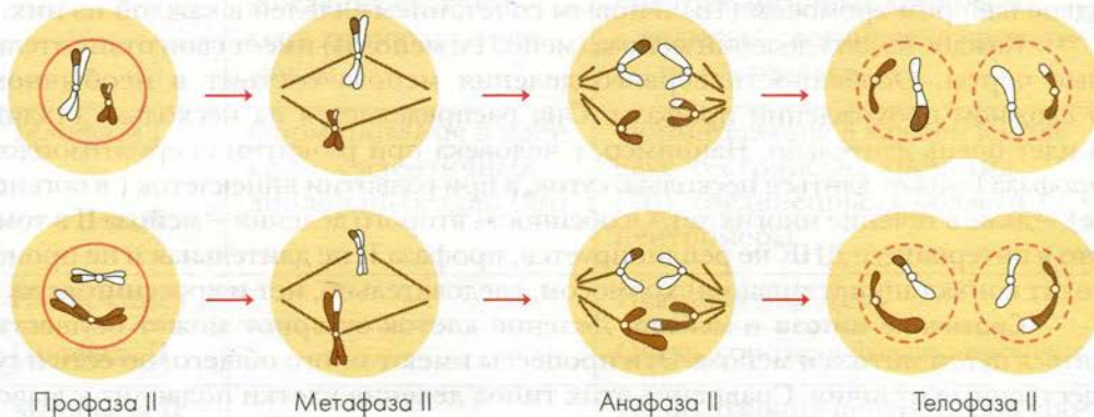
Рис. 42. Схема мейоза
