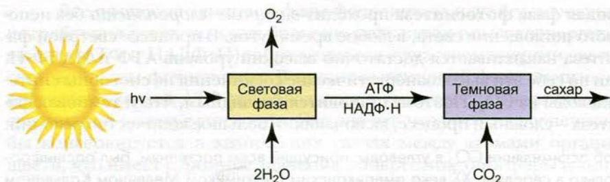
Рис. 62. Схема фотосинтеза
