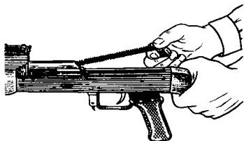
Рис. 52. Отделение возвратного механизма
