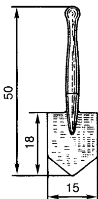
Рис. 60. Лопата малая
