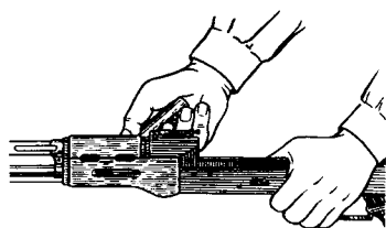
Рис. 55. Поворот замыкателя газовой трубки при помощи пеналя принадлежности
