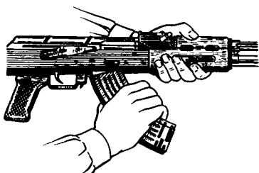
Рис. 57. Присоединение магазина
