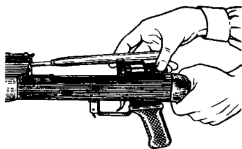
Рис. 53. Отделение затворной рамы с затвором
