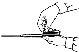
Рис. 54. Отделение затвора от затворной рамы
