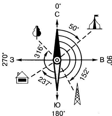
Рис. 6. Магнитные азимуты
